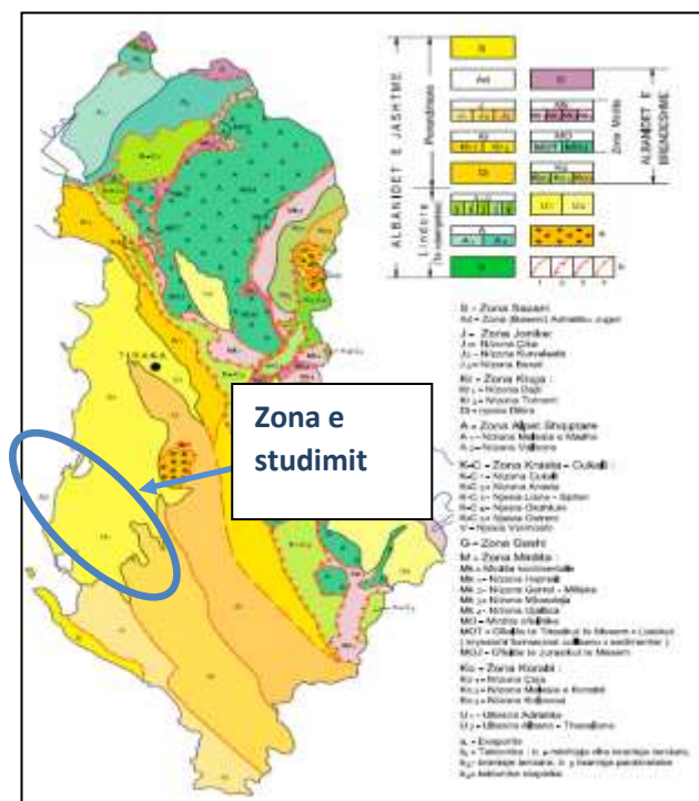
Harta tektonike e Shqipërisë (skematike)
