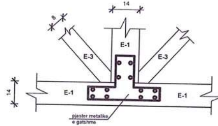
DETAJ D-2 SHK 1:20
