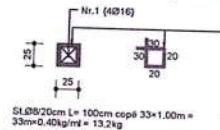
PRER. TIP E BR.2Ç SHK. 1:40
