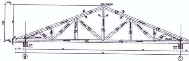
SKEMA E ELEMENTEVE TE KAPRIATES KAP-1
