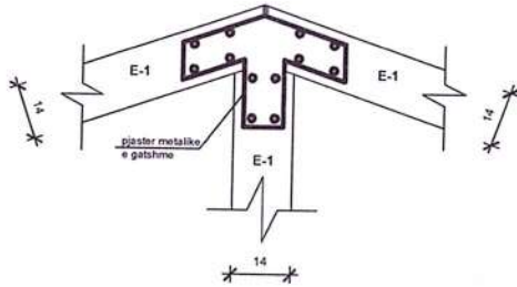
DETAJ D-1 SHK 1:20
