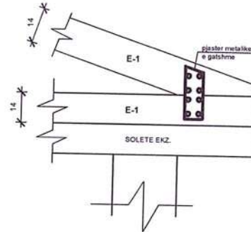
DETAJ D-3 SHK 1:20
