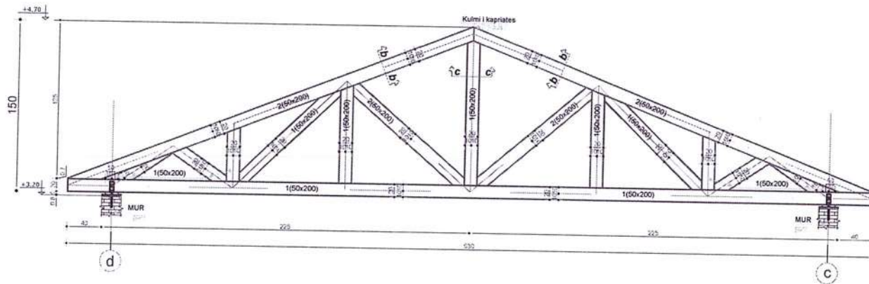
DETAJ D-1 SHK 1:20
