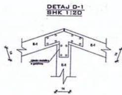
KULMI I KAPRIATES
