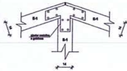
KULMI I KAPRIATES
