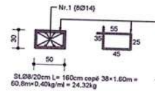
PRER. TIP E BR.1
