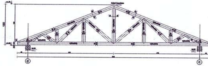
SHKEMA E ELEMENTEVE TE KAPRIATES KAP-1
