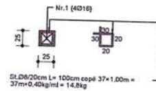
PRER. TIP E BR.1Ç
