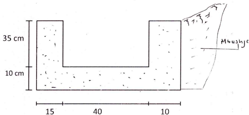
Detaji kanali Venisht (Lagjia Fejze) ,Beton C16/20
