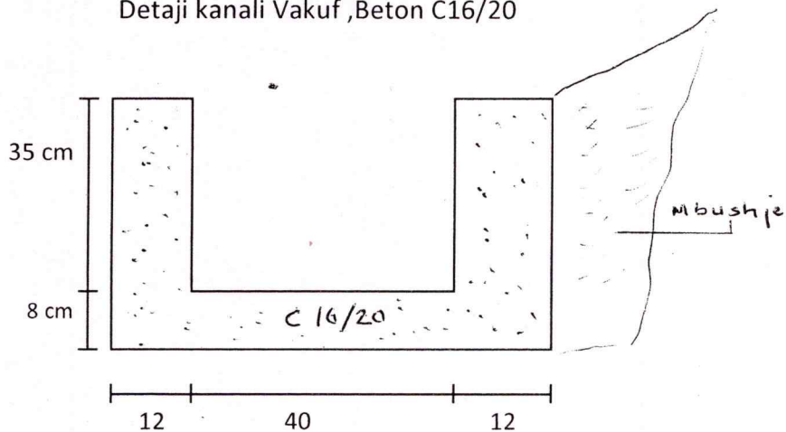
Detaji kanali Vakuf ,Beton C16/20
