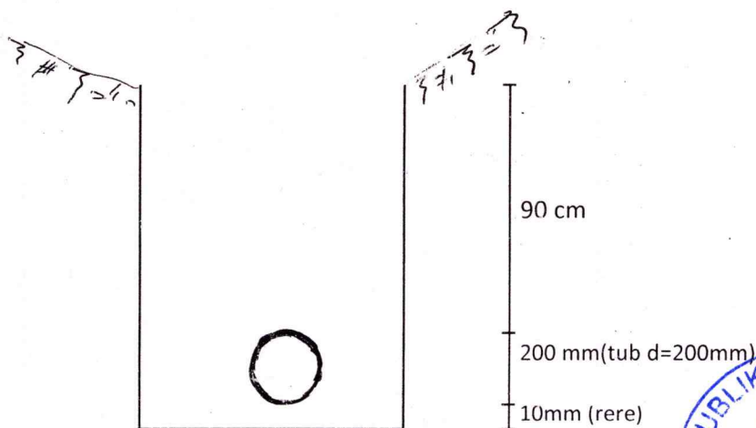
Detaji vendosje tubi HDPE (Venisht,Lagj.Fejze)
