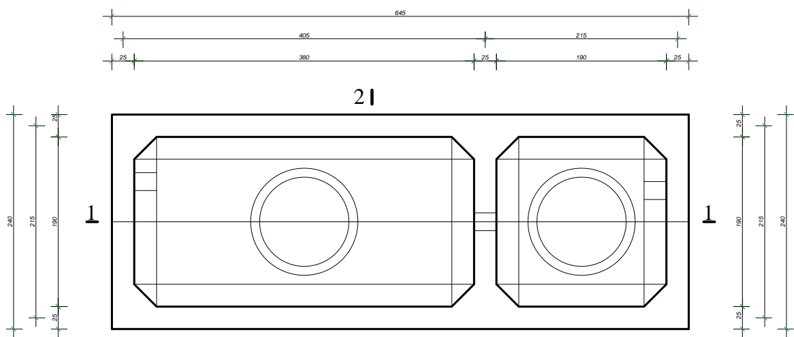
PLANIMETRIA SHK.1:50
