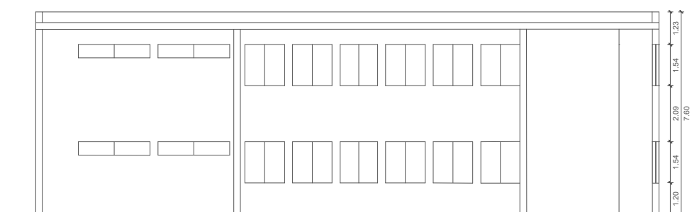
PRERJA A-A'
