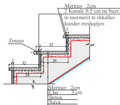
DETAJI I SHKALLEVE TE JASHTME
