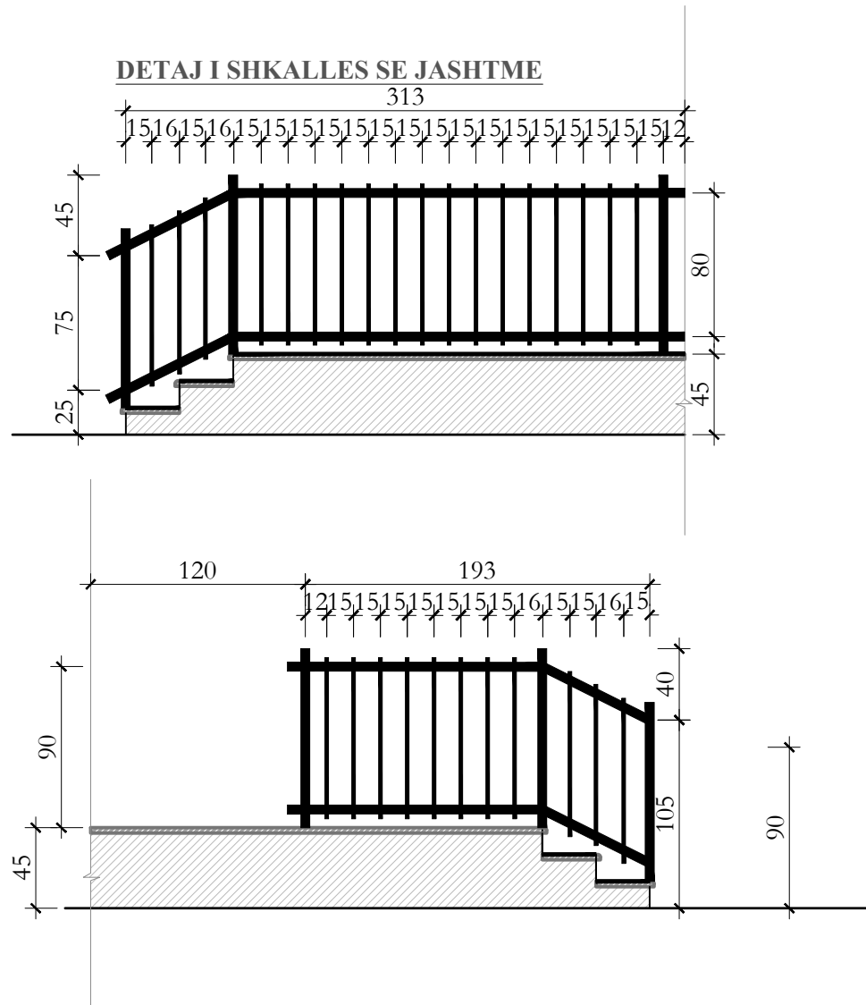
Detaj i shkalleve te jashtme SH-3
