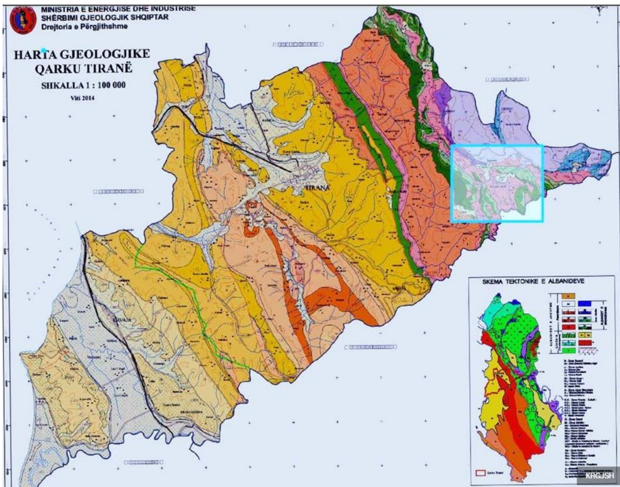
Figura 2 Struktura Gjeologjike e Qarkut te Tiranës
