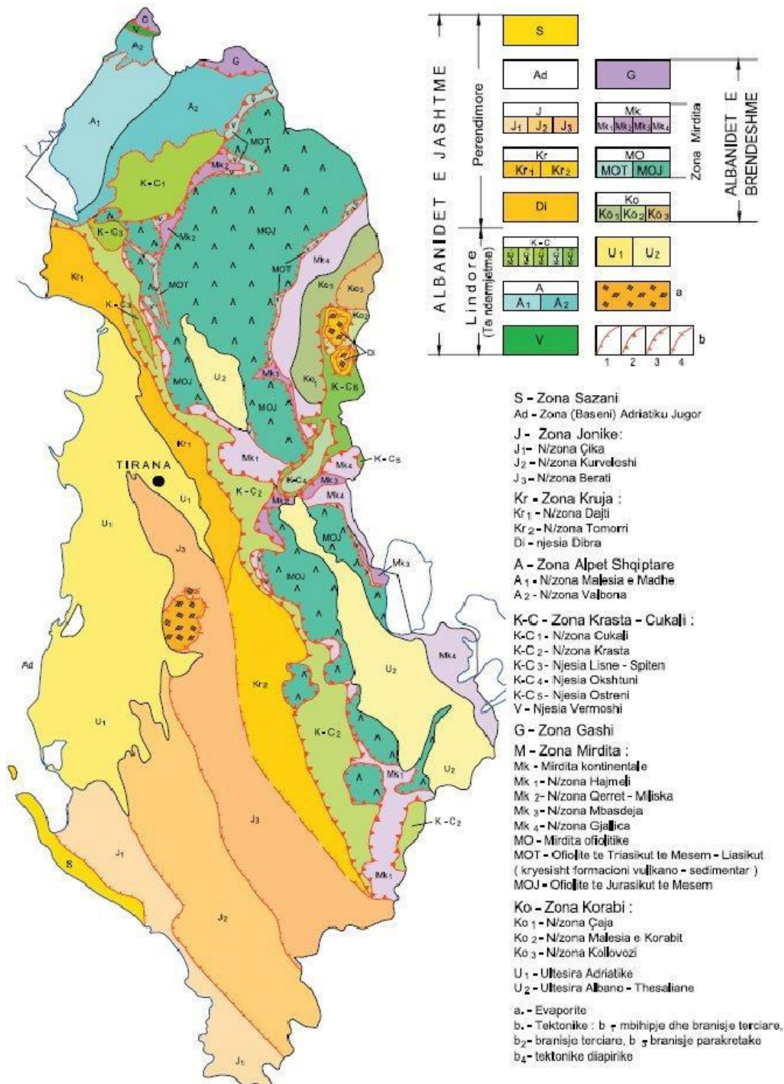
Figura 1 Struktura Gjeologjike e Shqipërisë
