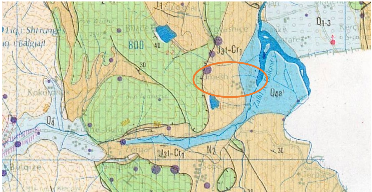
Fig. 16 – Pjese nga harta hidrogeologjike e Shqiperise me shkalle 1:200000
