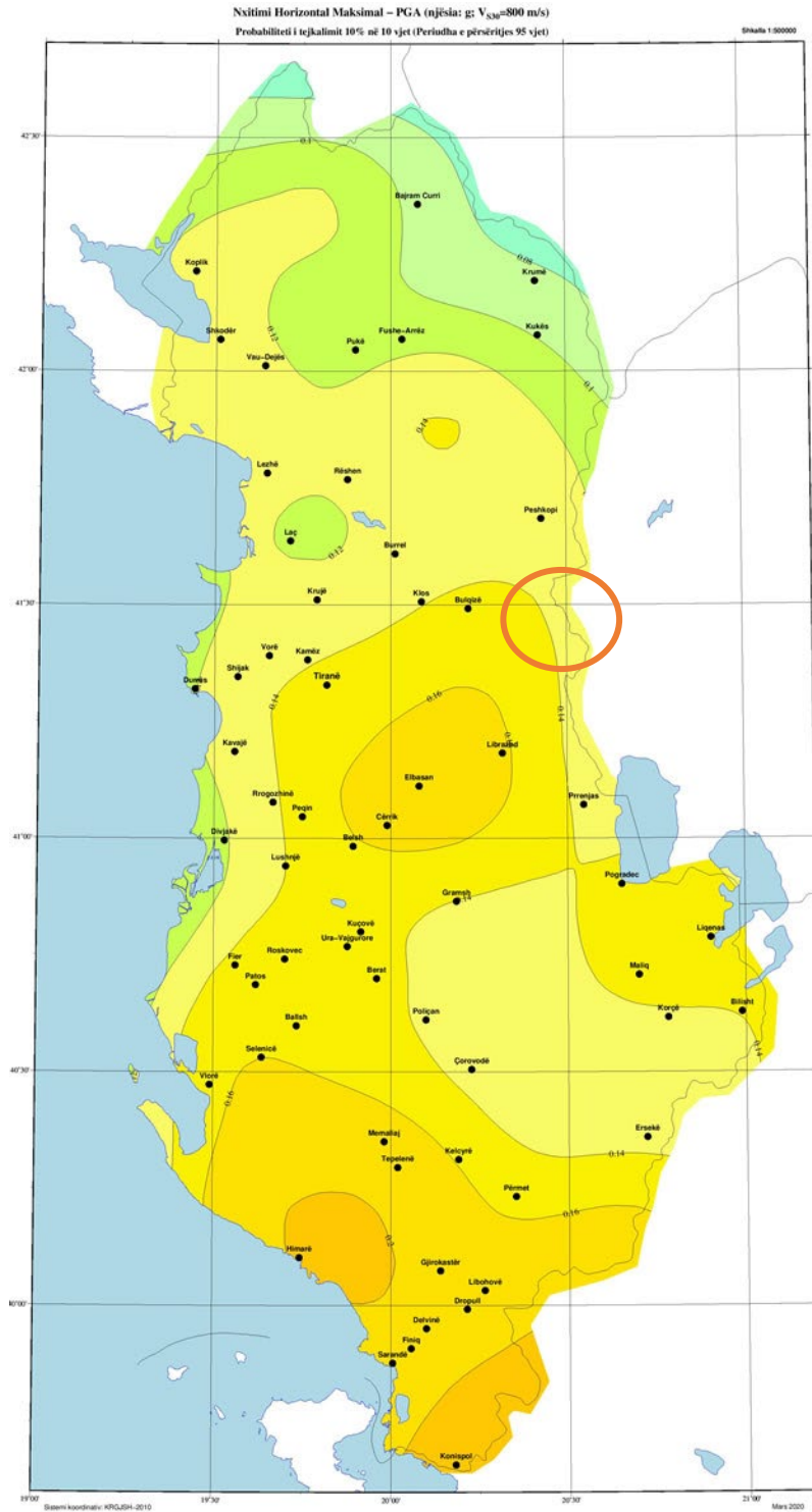
Fig. 10 – Harta e shpërndarjes së PGA për probabilitet tejkalimi 10% / 10 vjet (ose periudha përsëritje 95 vite)
