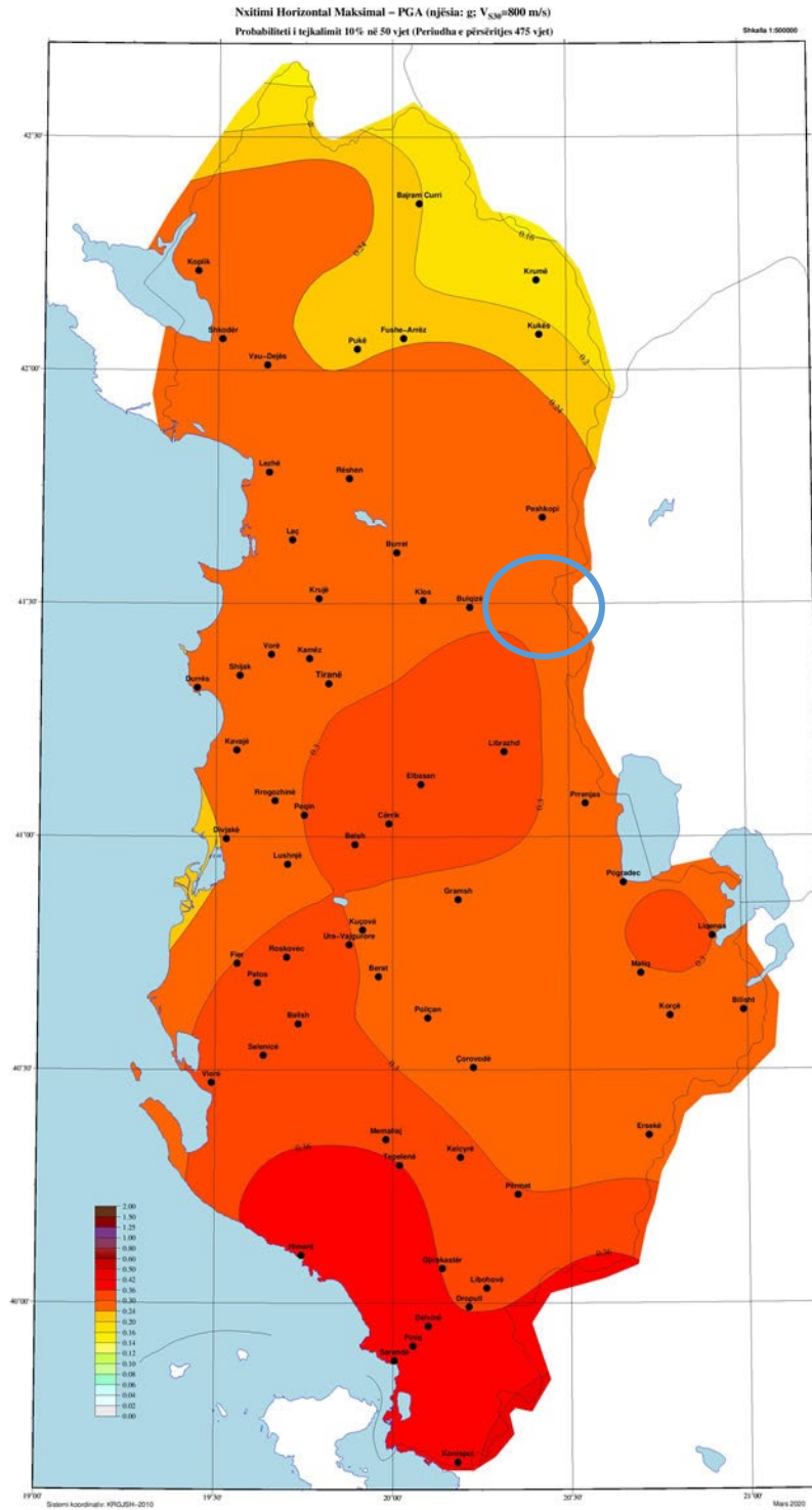
Fig. 11 – Harta e shpërndarjes së PGA për probabilitet tejkalimi 10% / 50 vjet (ose periudhe përsëritje 475 vite)
