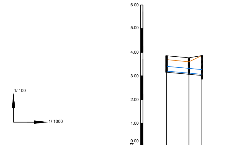
Profili Gjatësor, Puseta 6-5-P KUB (Pusete kryesore KUB), Sh.V.1:100
