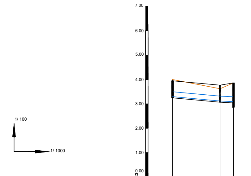
Profili Gjatësor, Puseta 4-5-P KUB (Pusete kryesore KUB), Sh.V.1:100
