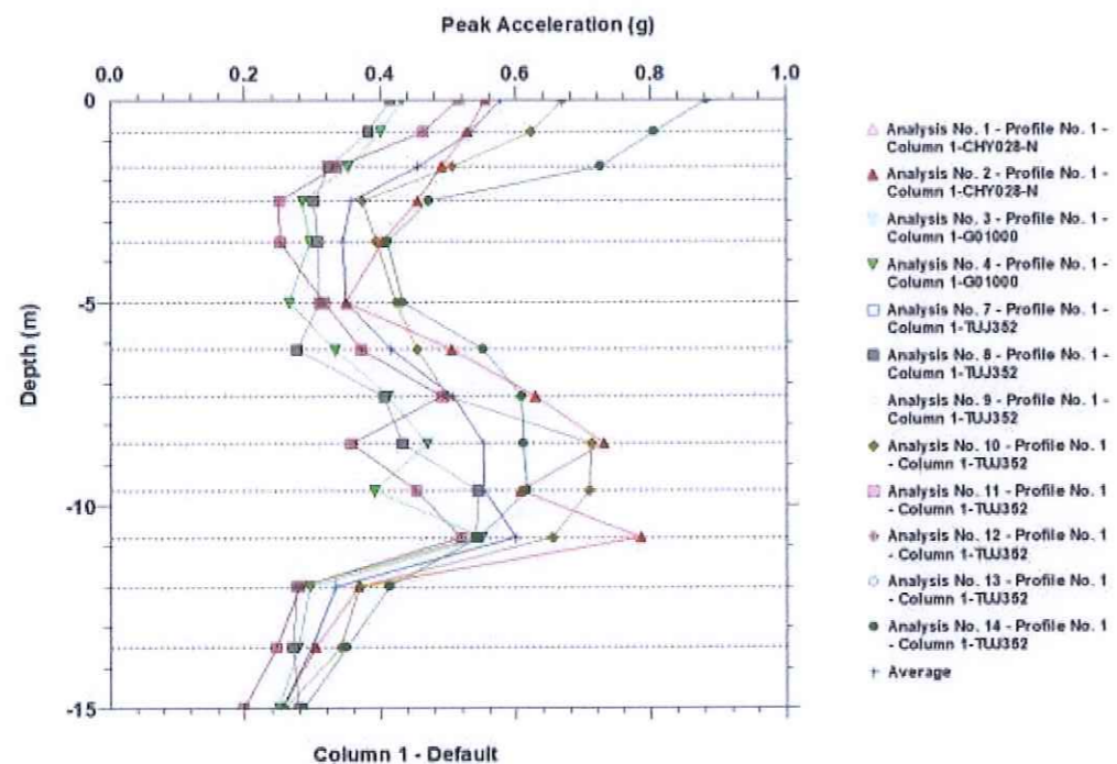
Fig. 5: Grafiku i ndryshimit te nxitimit maksimal nga shkembimi baze (thellesi 15.0 m) ne sipërfaqe te sheshit te ndertimit, llogaritur per periode perseritje 475 vjet me funksionet hyres te akselerogrameve te termeteve te lartpermendur, si dhe vlera e mesatarizuar e tyre (shih Tabelen 3).
