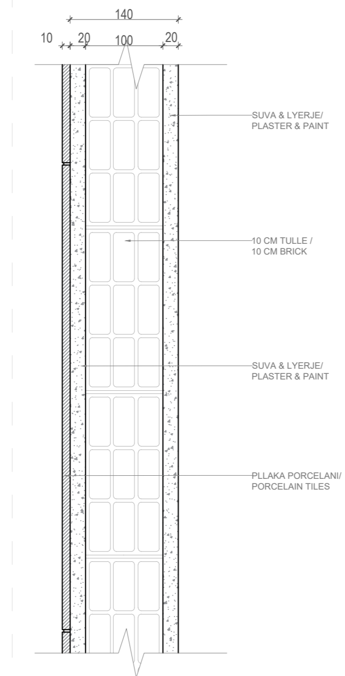
2 DETAIL TOILET WALL / DETAJ MUR TUALETI 1:5
