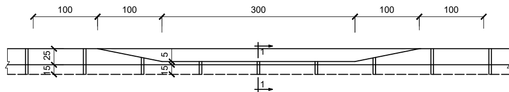
PRERJA A-A SHK.1:50
