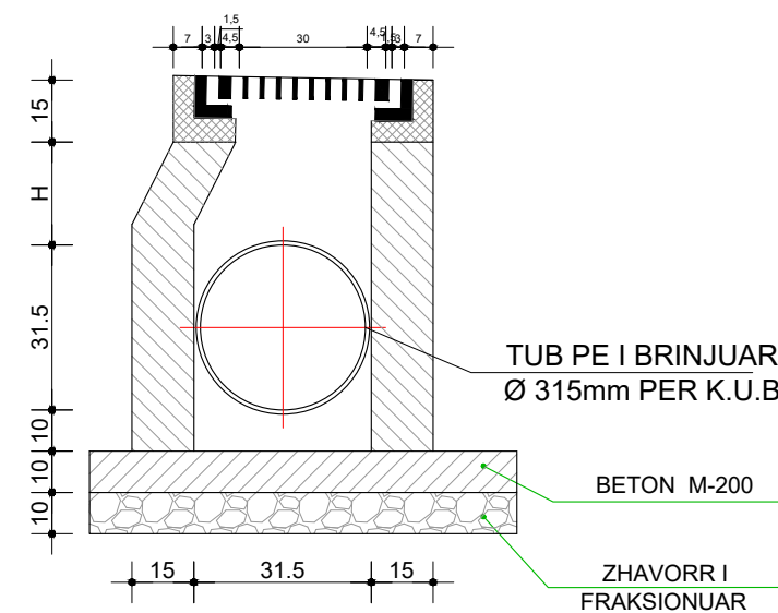
PRERJE B-B 1:20 (PER TUBA PE D=315 )
