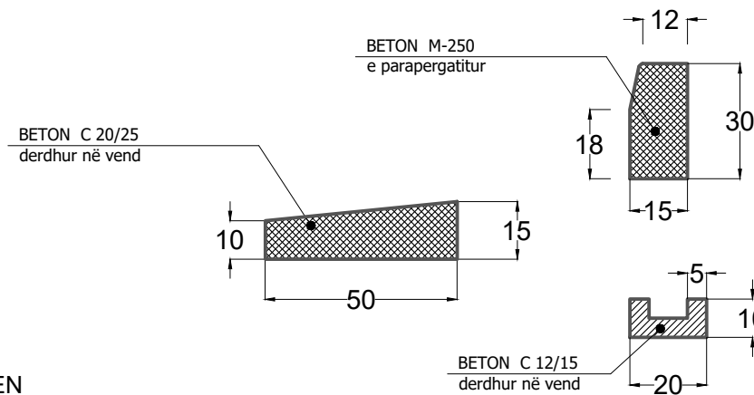
Detaji i Bordurës dhe kunetes Sh 1:15
