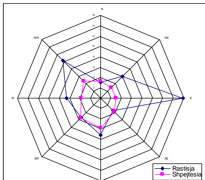
Fig. 4 Trendafili i erës për vlerat mesatare shumëvjeçare ne Vlore
