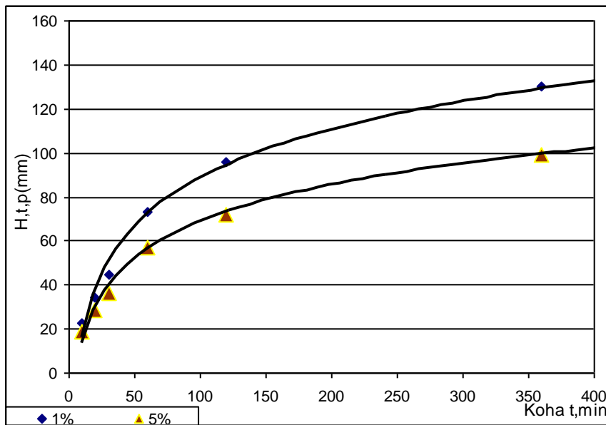
Fig. 6 Lakoret e varësisë së shtresës së shiut nga kohëzgjatja për probabilitet tejkalimi 1% dhe 5%
