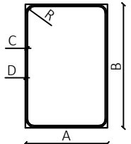
Shënjë kuadratike Skeda 2 "Drejtëkëndësh tregimi"
