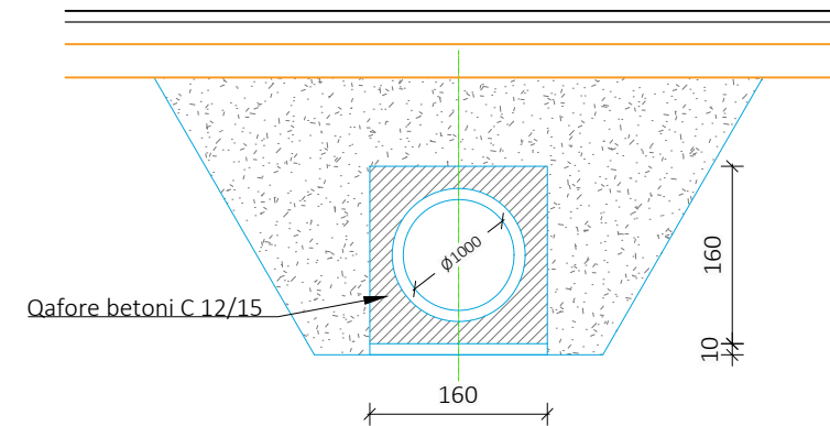
Prerje A-A
