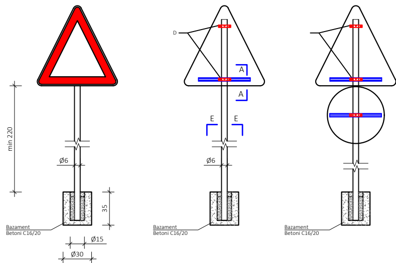
MENYRA E VENDOSJES SE TABELAVE RRUGORE SH 1:25
