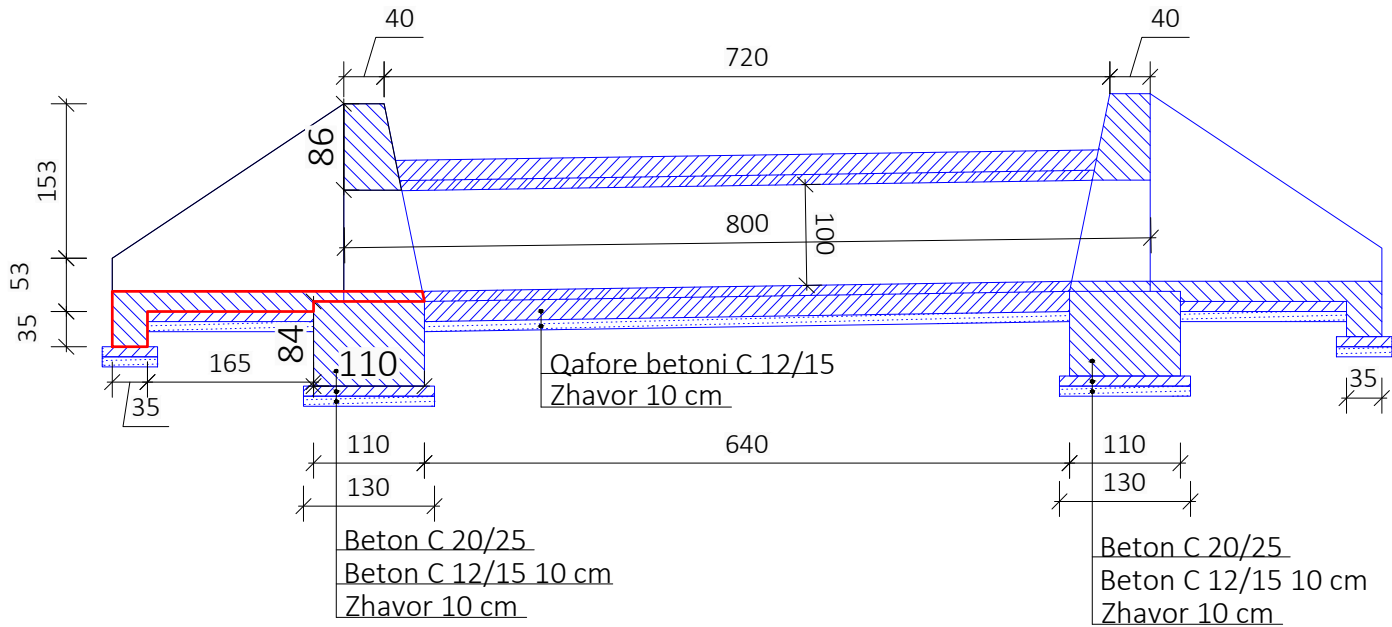
PRERJE GJATESORE E TOMBINOS B-B
