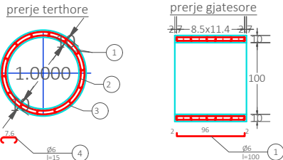
Armatura Spirale
