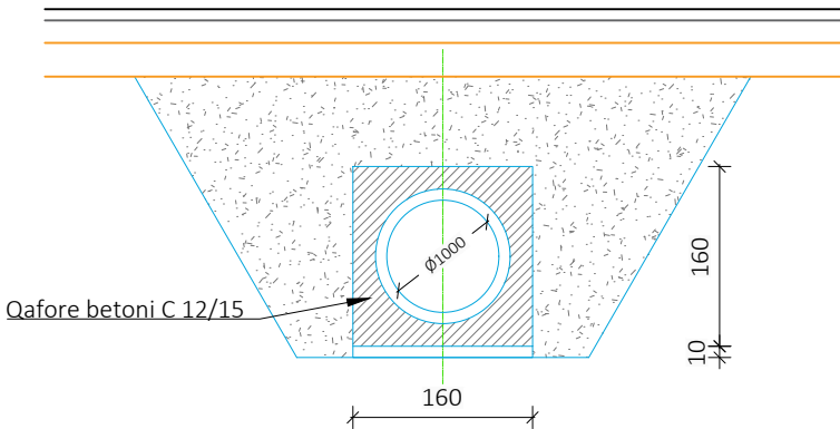
Prerje A-A
