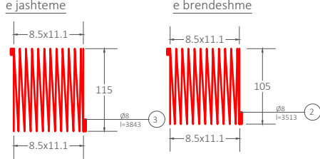
Armatura Spirale
