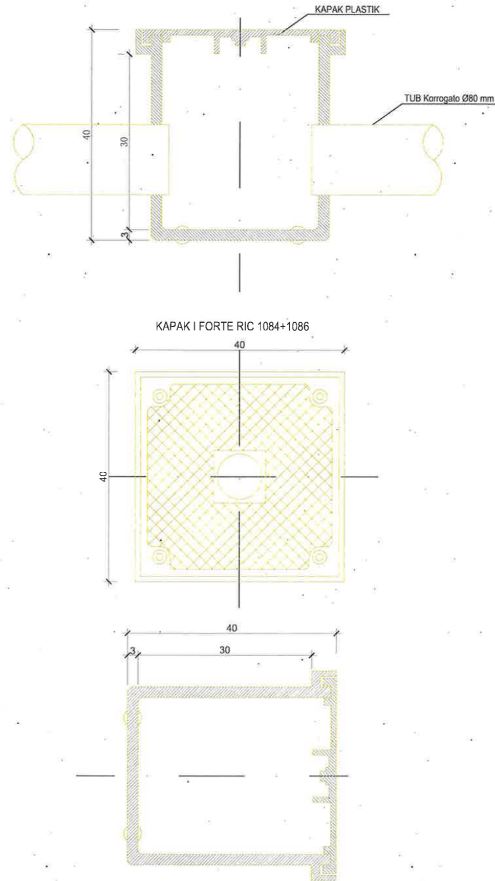
PLANI I DETAJIT TE PUSETES ,PLASTIKE 40X40X40 CM, SE NDRICIMIT DHE I MONTIMIT TE SAJ NE TOKE ME TUB
