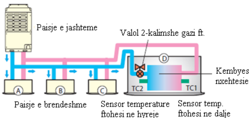
Fig.2 Skema pricipiale e sistemit VRF
