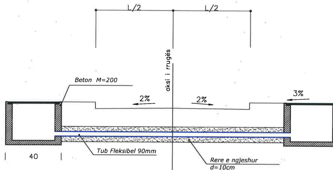
Prerje e vendosjes së pusetave
