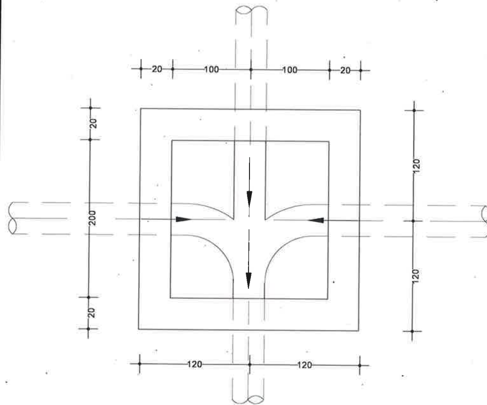
PLANIMETRIA E HYRJES NE PUSETE SH. 1 / 20
