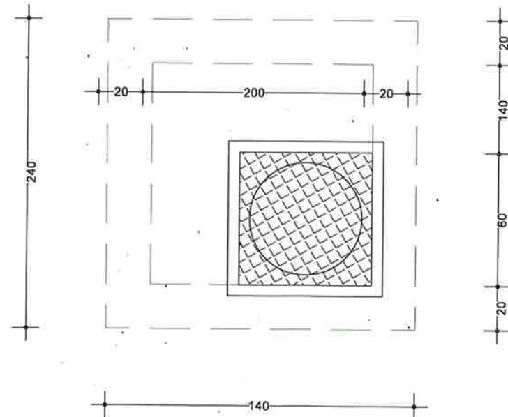
PLANIMETRIA E HYRJES NE PUSETE SH. 1 / 20
