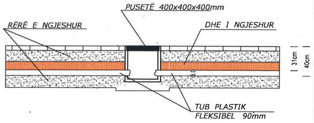
Hollësi e vendosjes së pusetës per Tub fleksibel 90mm
