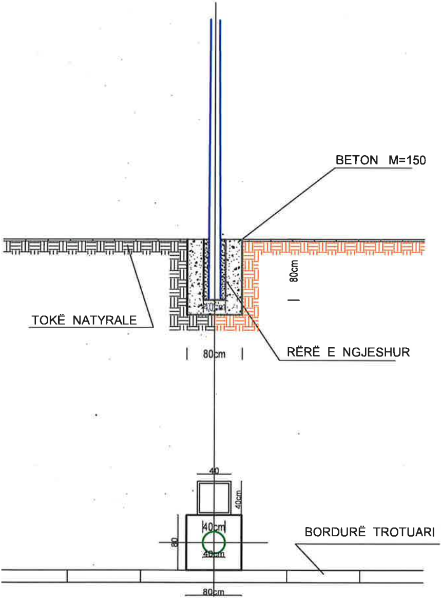
Hollësi e inkastrimit të kolonës së ndriçuesit me lartësi H=9m
