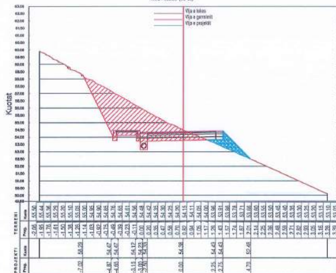
Km 0+350.00 (CS-39)
