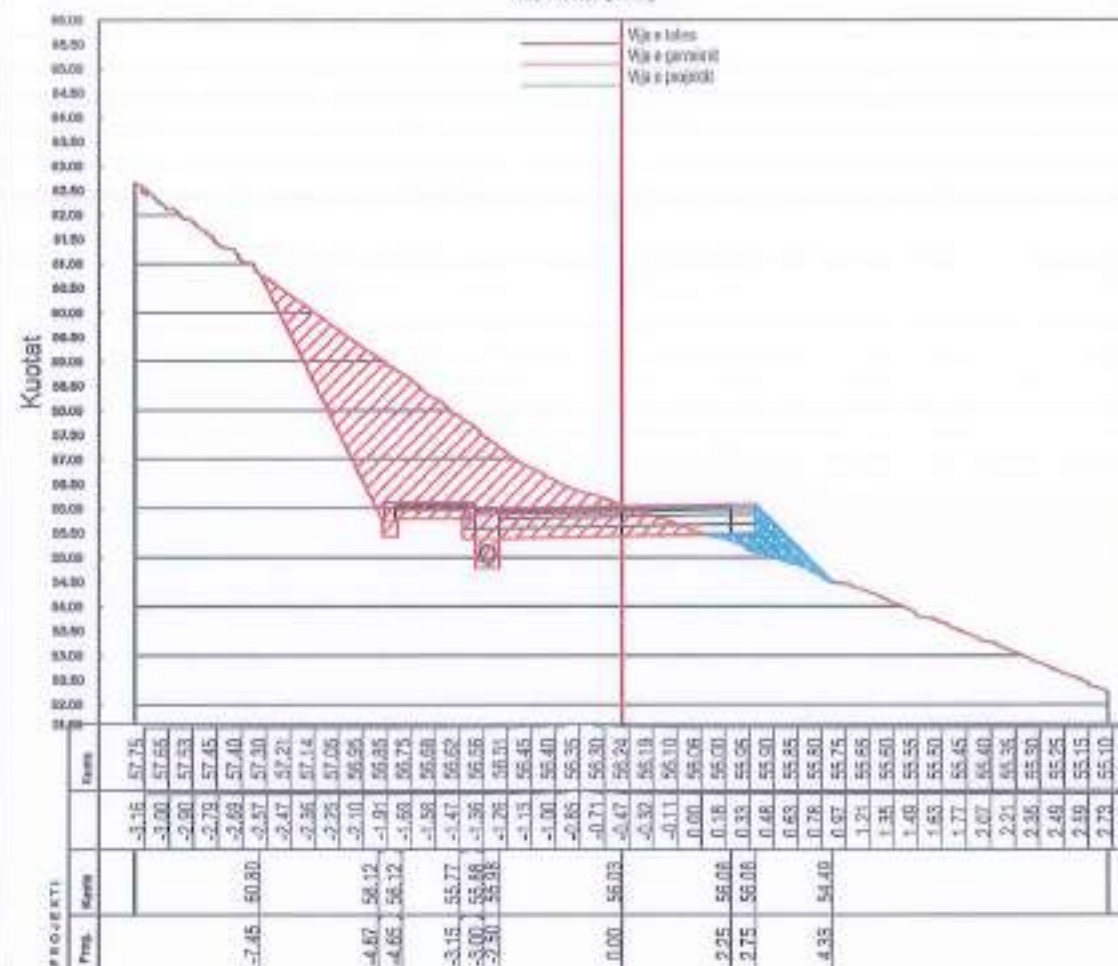
Km 0+305.00 (CS-38)
