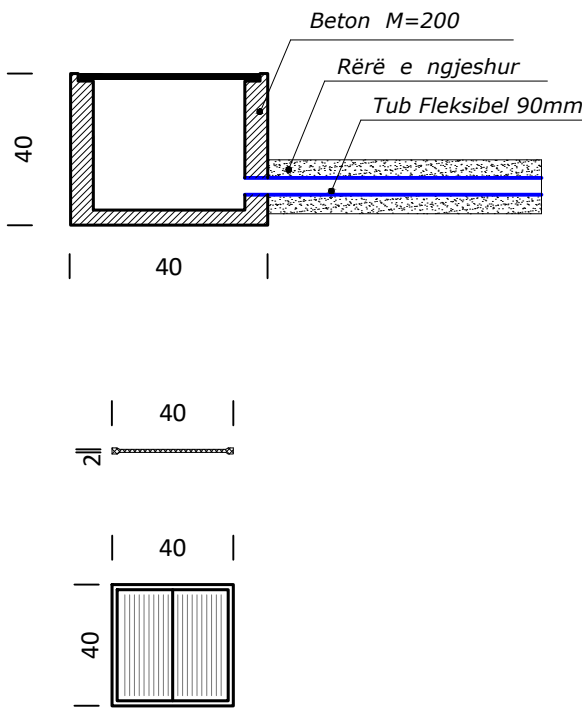
Kapaku i pusetës prej gize
