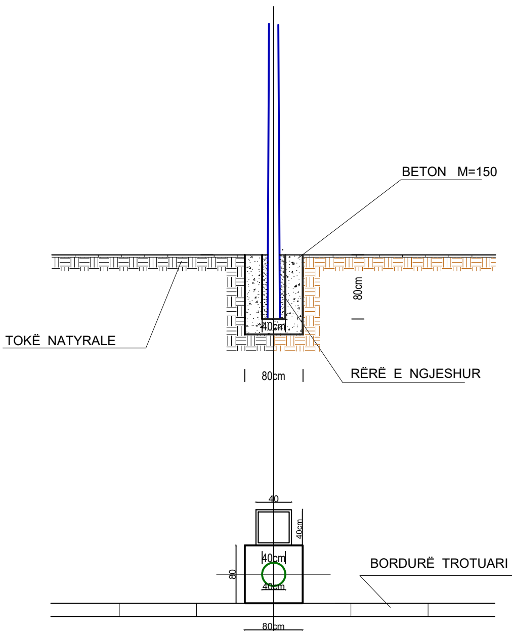
Hollësi e inkastrimit të kolonës së ndriçuesit me lartësi H=7.8m
