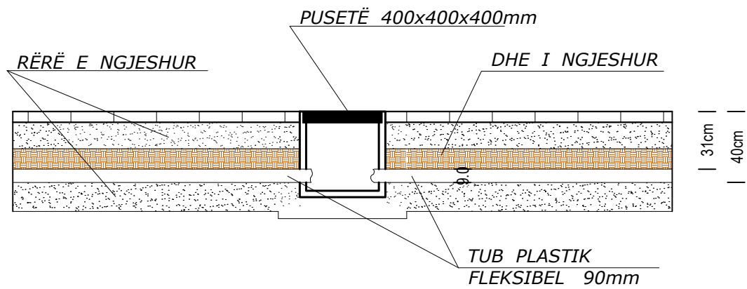
Hollësi e vendosjes së pusetës per Tub metalik 110mm
