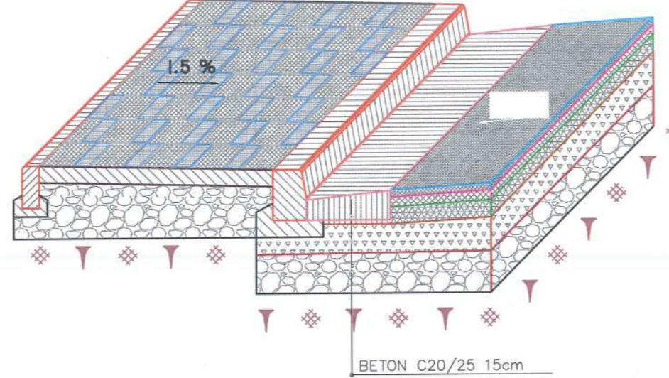
PAMJE E BORDURAVE DHE TROTUARIT
