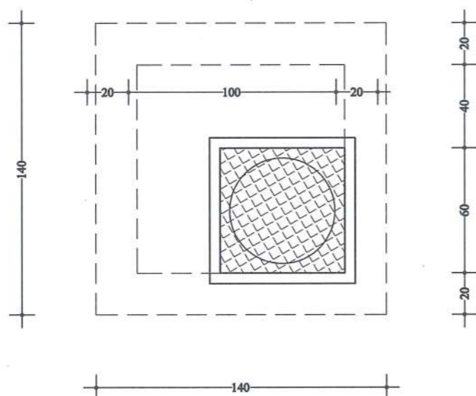
PLANIMETRIA E HYRJES NE PUSETE SH. 1 / 25
