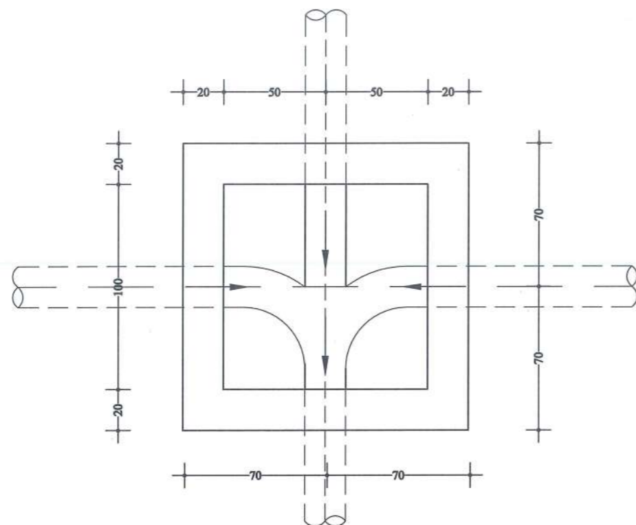
PLANIMETRIA E HYRJES NE PUSETE SH. 1 / 25
