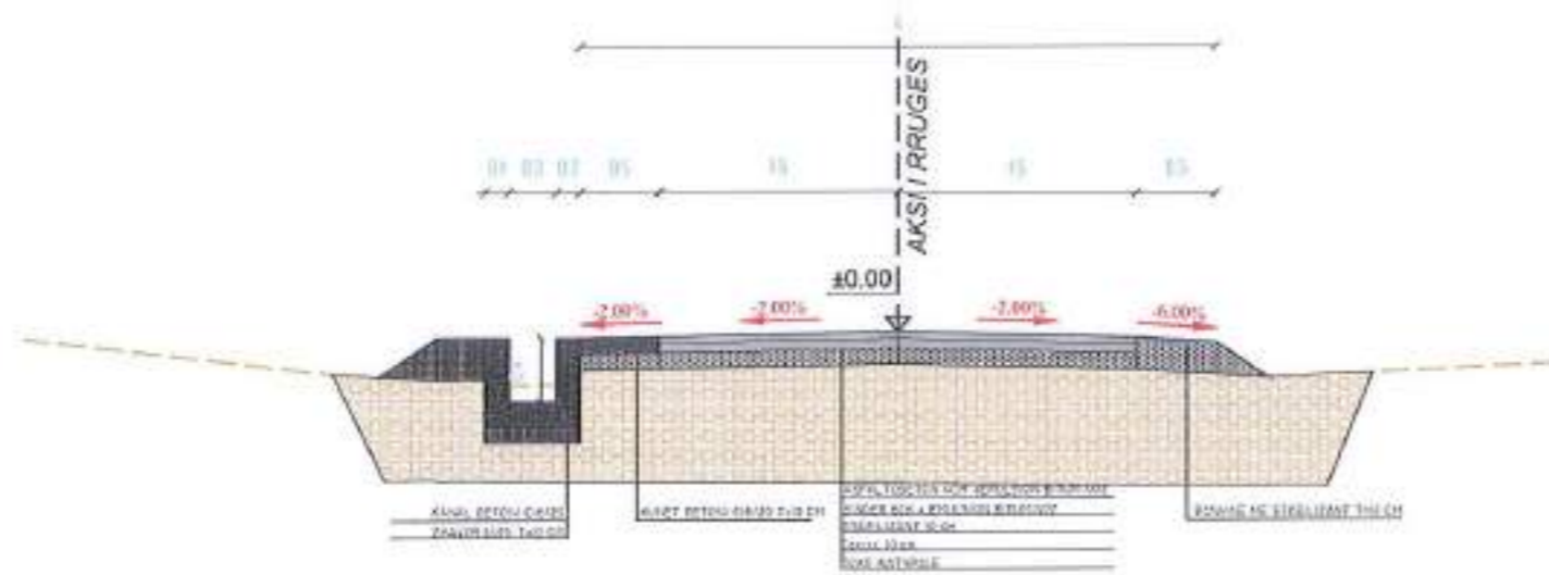
Profilë tërthor tip 1 i rruges kryesore Km 0+000- Km 0+240
