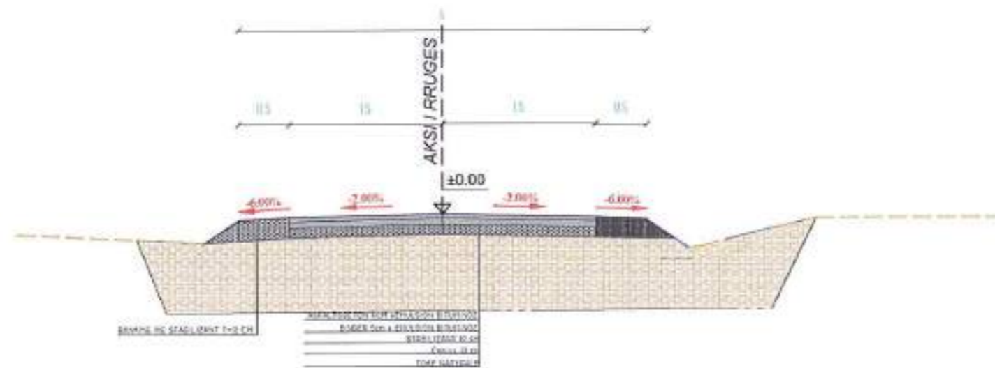
Profilë tërthor tip 2 i rruges kryesore Km 0+240 - Km 0+550
