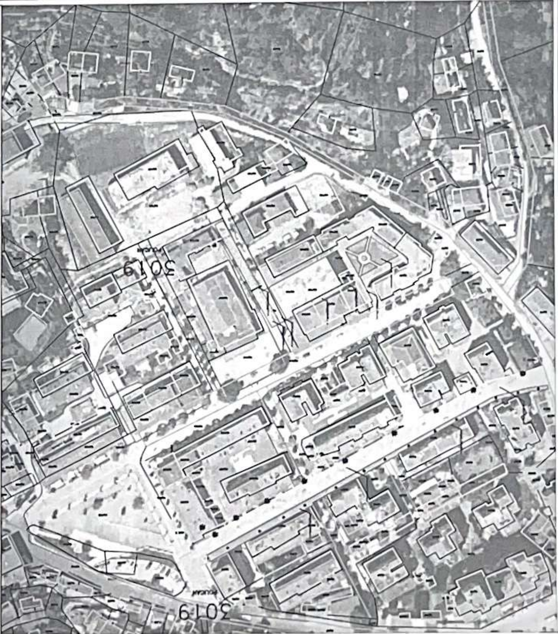
Plani i Vendosjes ne raport me Qytetin Sh. 1:2500
