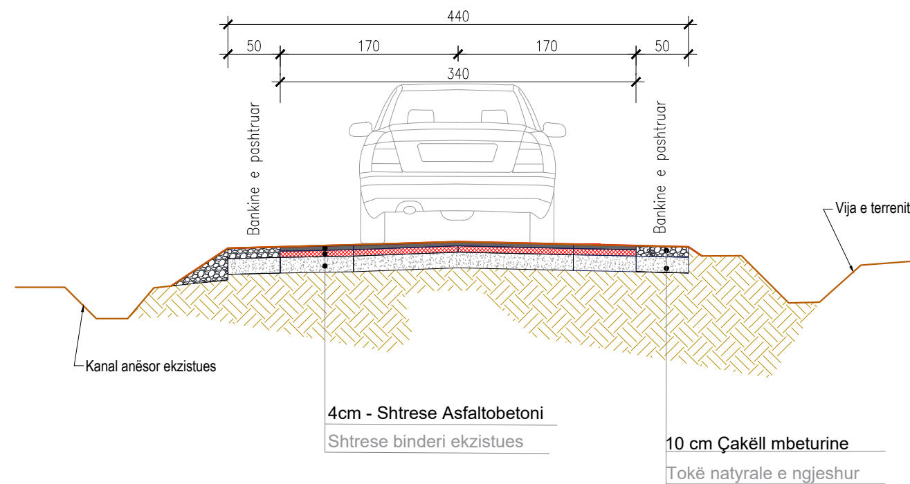
SEKSIONI TERHOT TIP 2 (RIVESHJE) PK.3-PK.4, PK.5-PK.6, PK.7-PK.8
