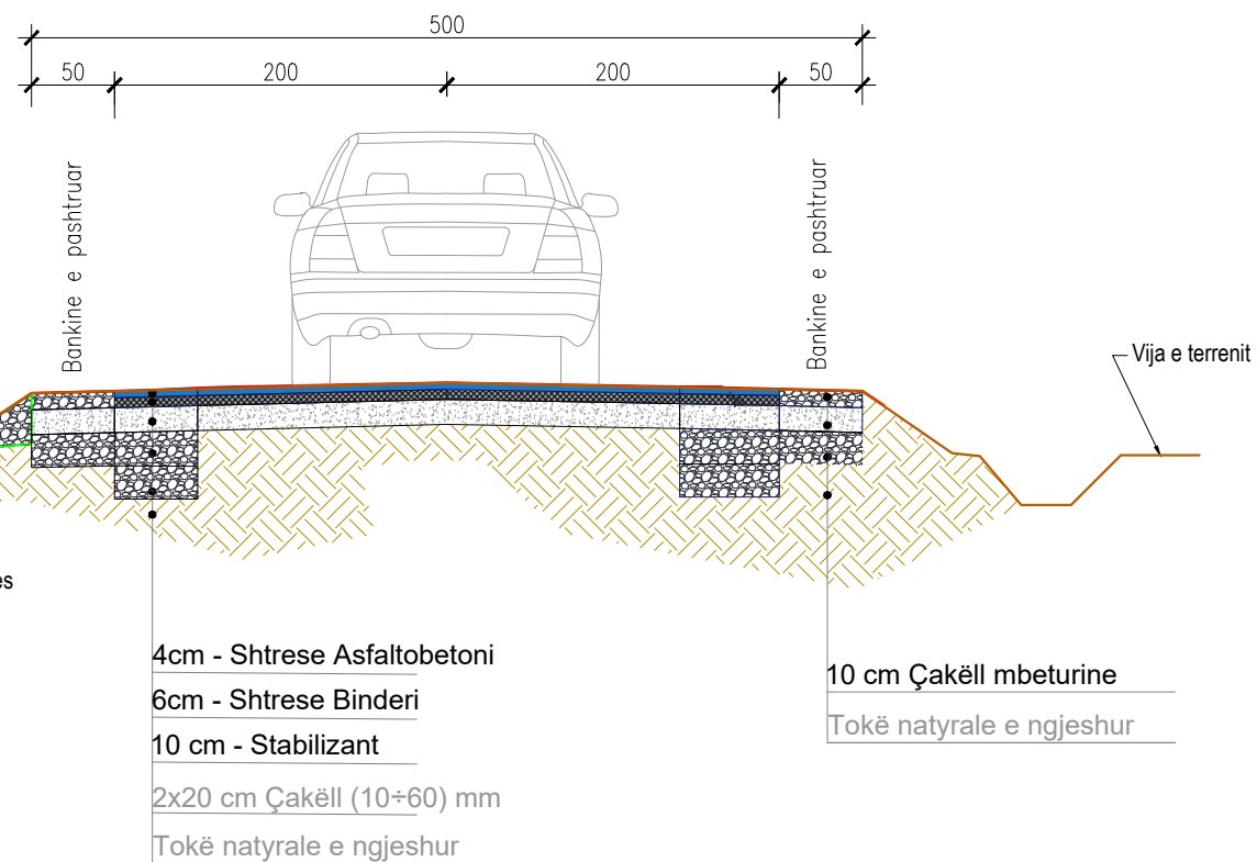
SEKSIONI TERTHOR TIP (ASFALT I RI) PK.1-PK.2
