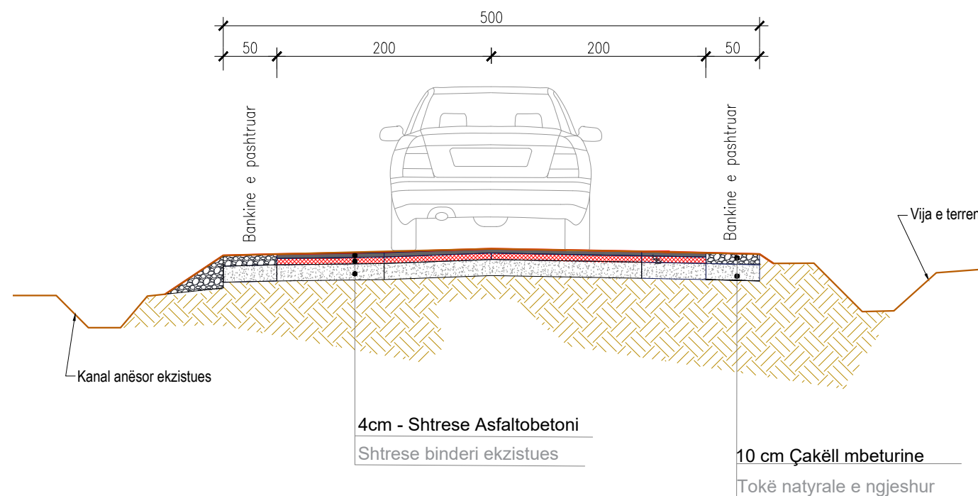
SEKSIONI TERTHOT TIP 2 (RIVESHJE) PK.2-PK.3
