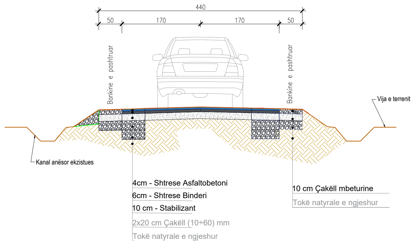
SEKSIONI TERTHOR TIP (ASFALT I RI) PK.4-PK.5, PK.6-PK.7
