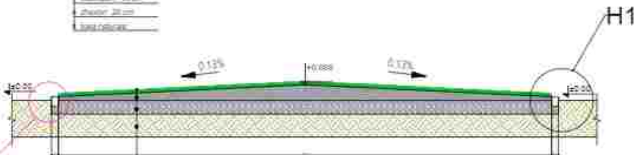
PRERJA B
