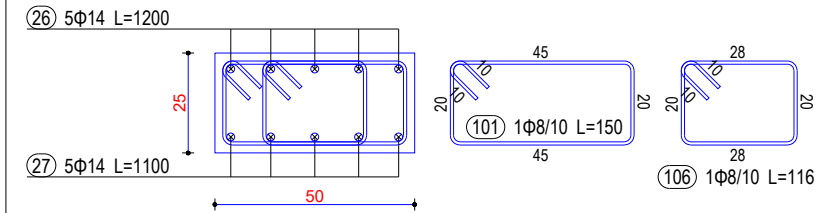
Seksioni 3-3
