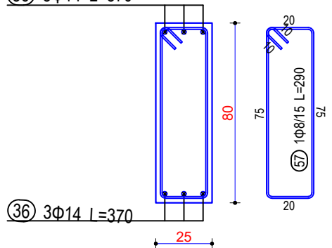
Seksioni 5-5
