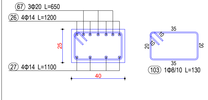
Seksioni 1-1
