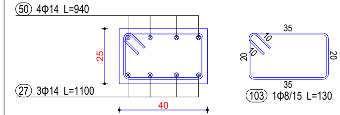
Seksioni 2-2
