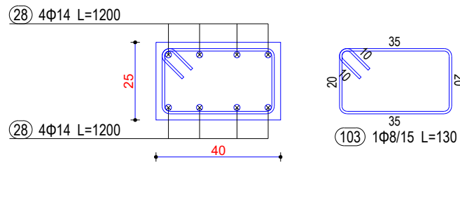
Seksioni 6-6
