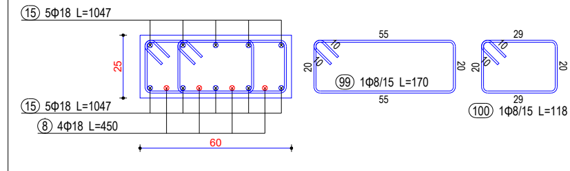
Seksioni 4-4
