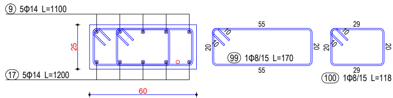
Seksioni 9-9
