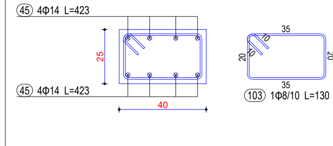
Seksioni 12-12
