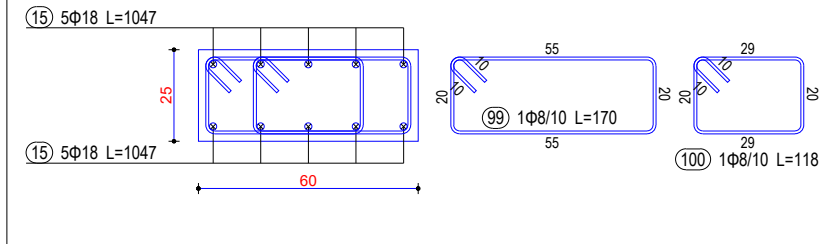
Seksioni 5-5
