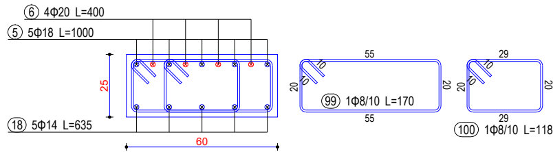
Seksioni 15-15
