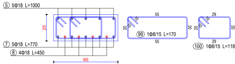
Seksioni 17-17
