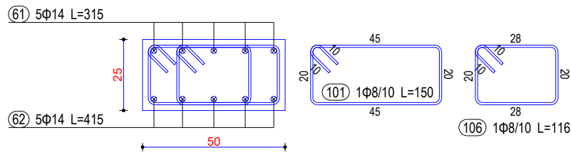
Seksioni 3-3
