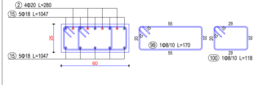
Seksioni 1-1
