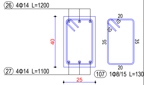
Seksioni 2-2
