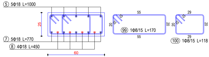
Seksioni 2-2
