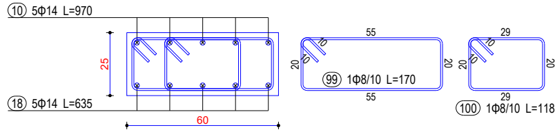
Seksioni 13-13
