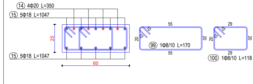
Seksioni 4-4
