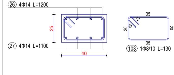
Seksioni 3-3
