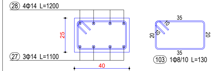
Seksioni 4-4
