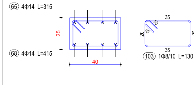
Seksioni 6-6
