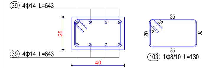
Seksioni 1-1
