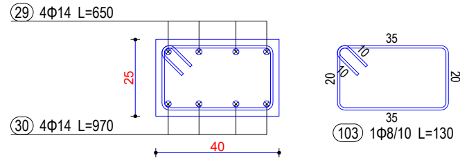
Seksioni 8-8
