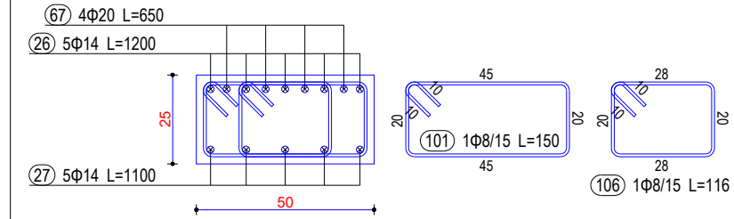
Seksioni 2-2
