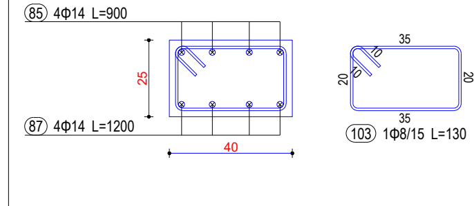
Seksioni 4-4
