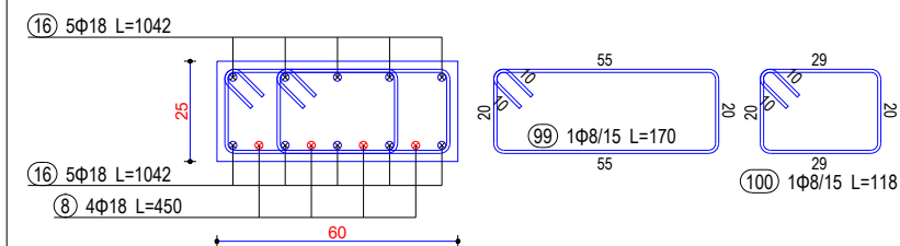
Seksioni 3-3
