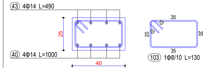
Seksioni 5-5
