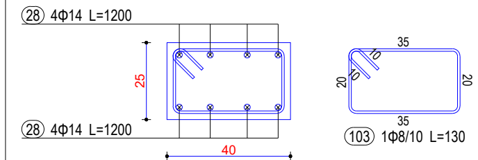
Seksioni 5-5
