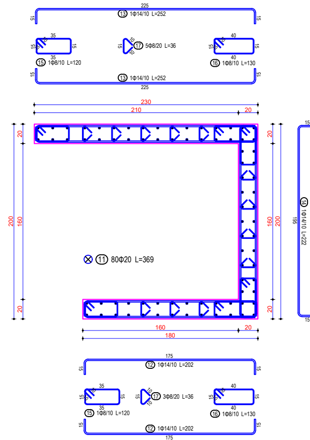
Seksioni 2-2
