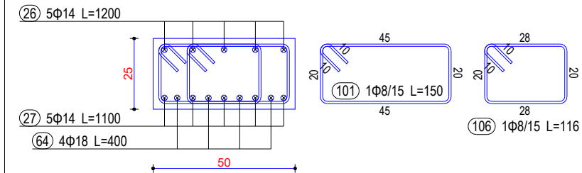
Seksioni 3-3
