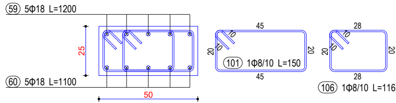
Seksioni 1-1
