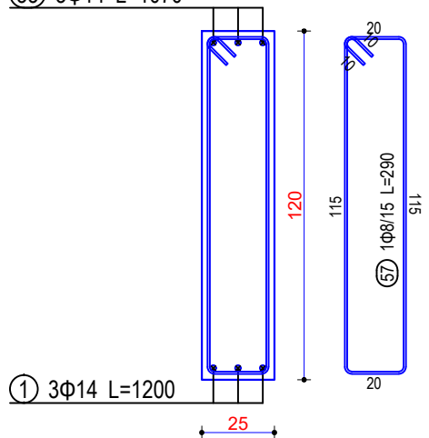
Seksioni 1-1
