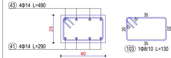
Seksioni 3-3
