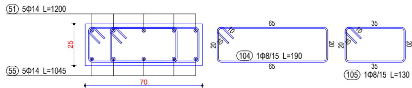
Seksioni 13-13
