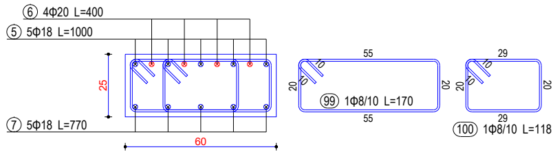
Seksioni 3-3
