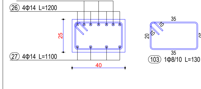
Seksioni 4-4
