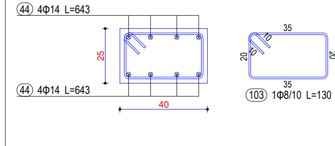
Seksioni 10-10
