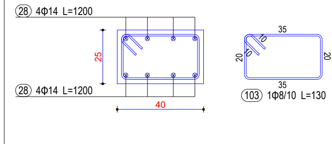
Seksioni 5-5
