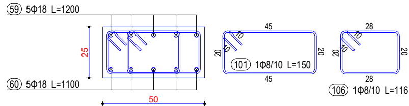
Seksioni 2-2
