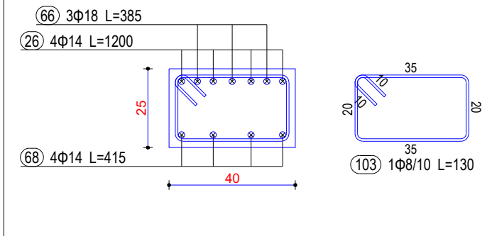
Seksioni 5-5
