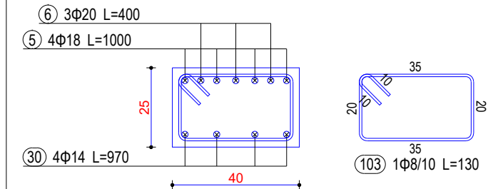
Seksioni 11-11
