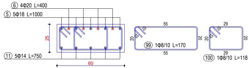
Seksioni 4-4
