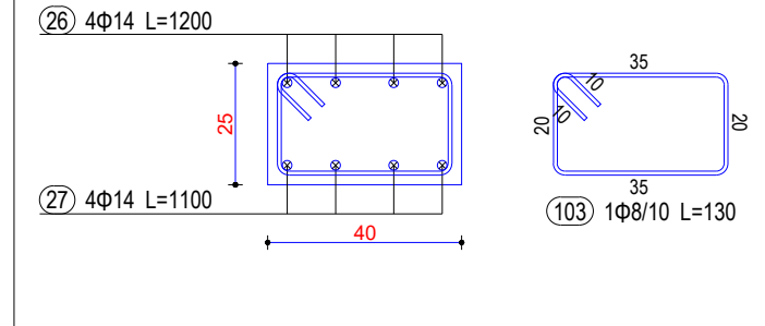
Seksioni 4-4
