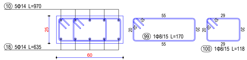
Seksioni 12-12
