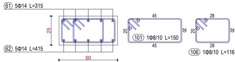
Seksioni 4-4
