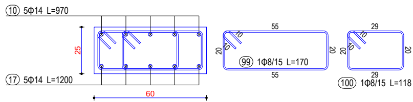
Seksioni 11-11
