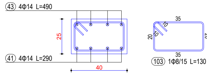
Seksioni 4-4
