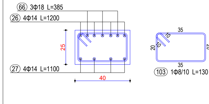
Seksioni 4-4
