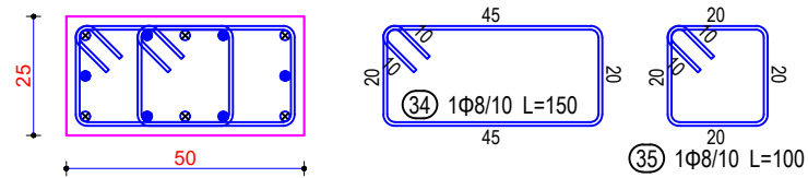
Seksioni 2-2
