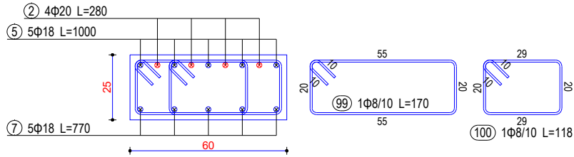
Seksioni 1-1
