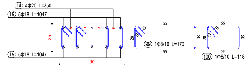
Seksioni 3-3
