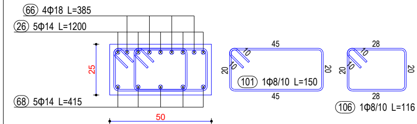
Seksioni 5-5
