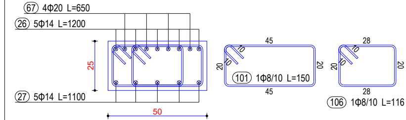
Seksioni 2-2
