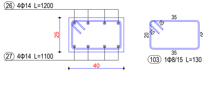
Seksioni 4-4
