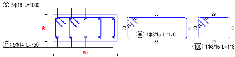
Seksioni 5-5
