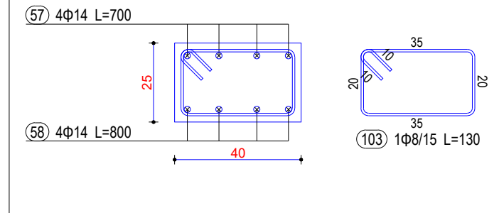
Seksioni 3-3
