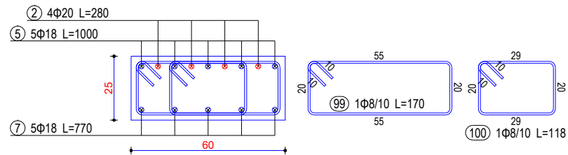
Seksioni 18-18
