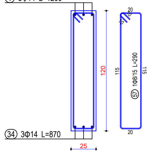
Seksioni 3-3
