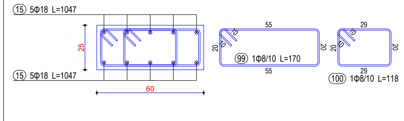
Seksioni 5-5
