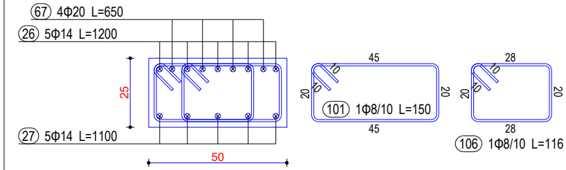
Seksioni 1-1
