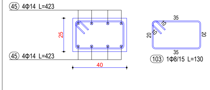
Seksioni 11-11
