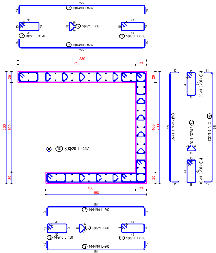
Seksioni 1-1
