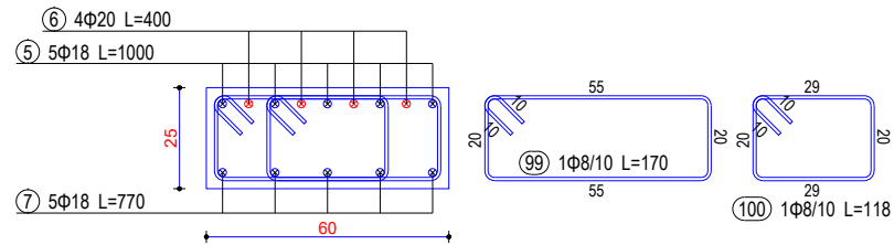
Seksioni 16-16
