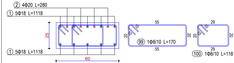
Seksioni 1-1
