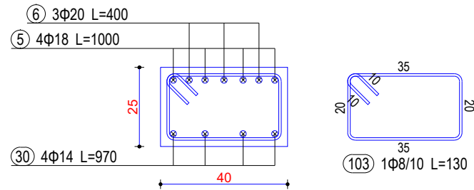
Seksioni 10-10
