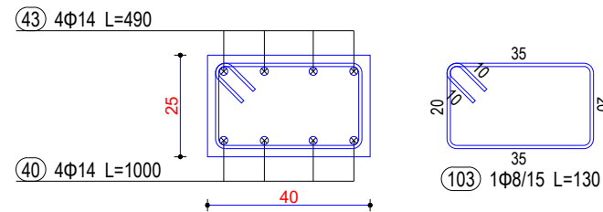
Seksioni 6-6
