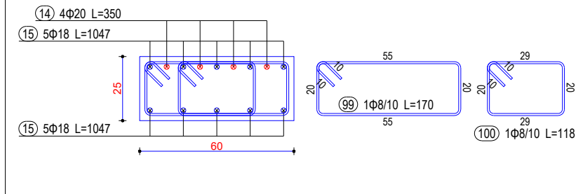
Seksioni 3-3
