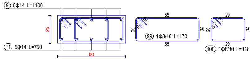
Seksioni 6-6
