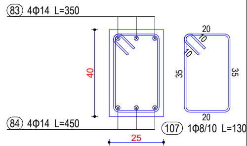
Seksioni 5-5
