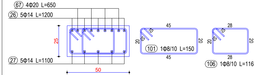
Seksioni 1-1
