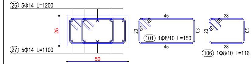
Seksioni 4-4
