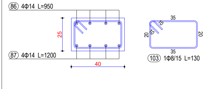
Seksioni 5-5
