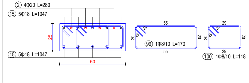
Seksioni 1-1
