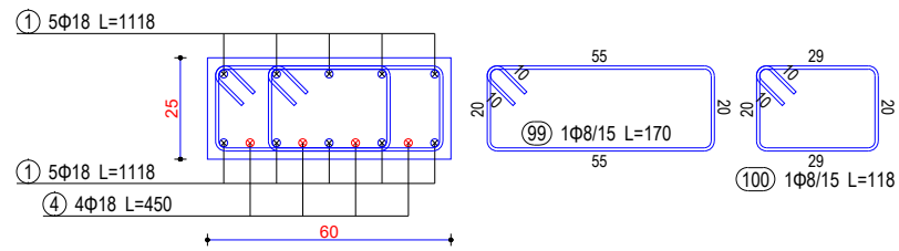
Seksioni 2-2
