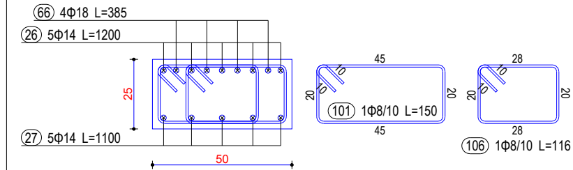
Seksioni 4-4
