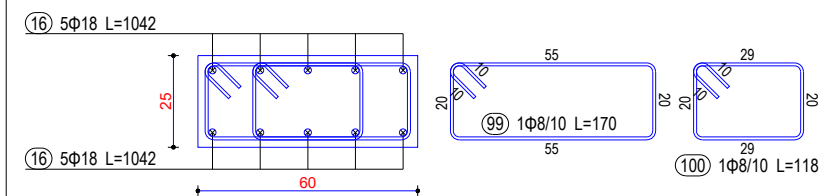
Seksioni 1-1
