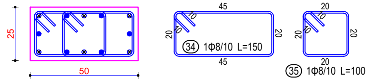
Seksioni 1-1
