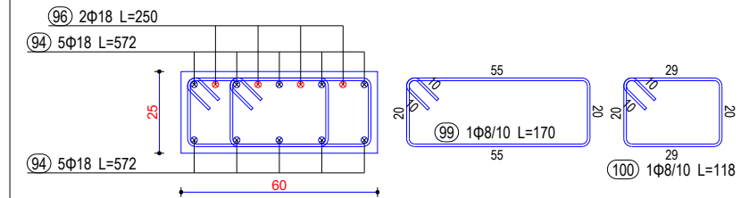
Seksioni 8-8
