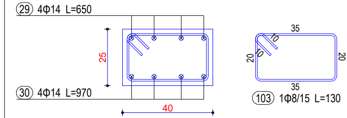
Seksioni 7-7
