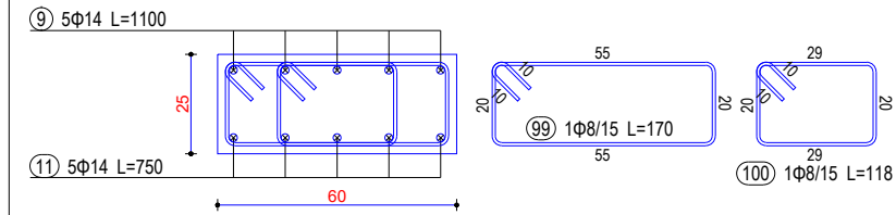
Seksioni 7-7
