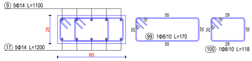
Seksioni 8-8
