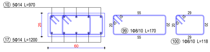
Seksioni 10-10
