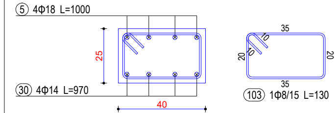
Seksioni 9-9
