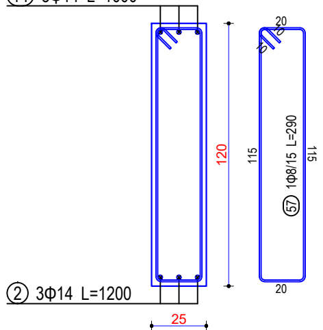
Seksioni 2-2
