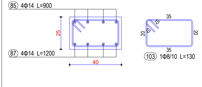
Seksioni 3-3
