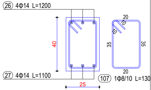
Seksioni 1-1
