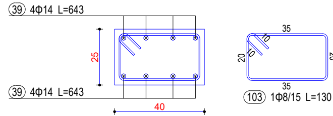
Seksioni 2-2
