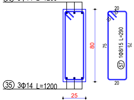
Seksioni 4-4
