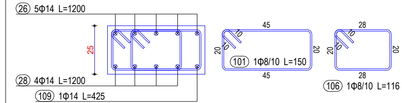
Seksioni 6-6
