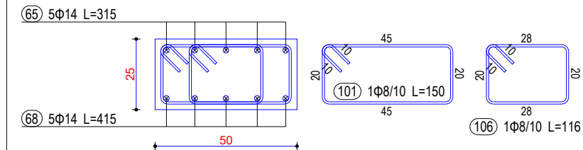
Seksioni 6-6
