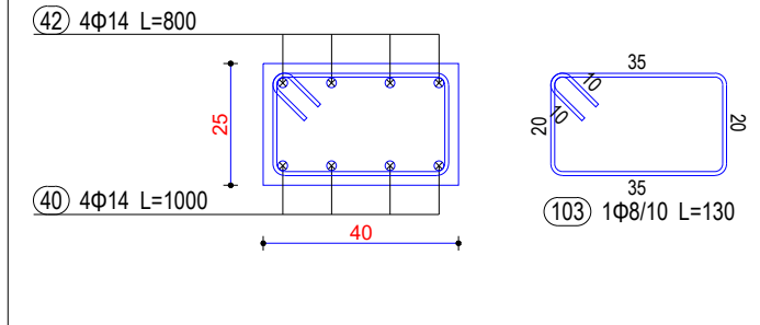
Seksioni 9-9
