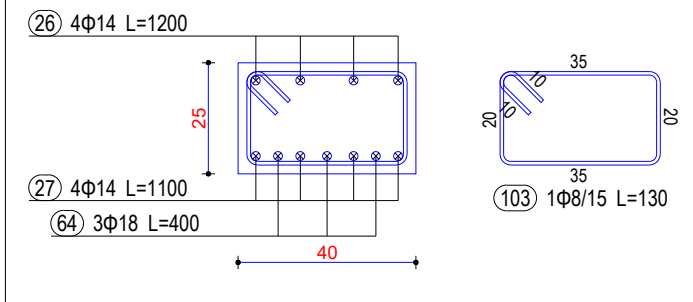
Seksioni 5-5
