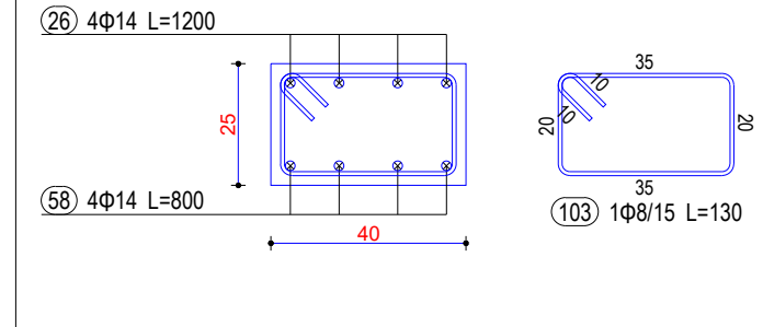
Seksioni 5-5
