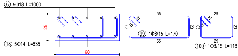
Seksioni 14-14
