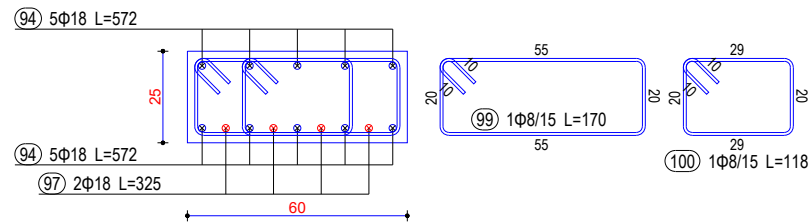
Seksioni 7-7
