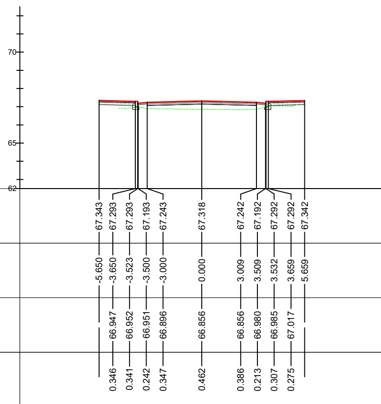
Chainage 20.000 Al-4
