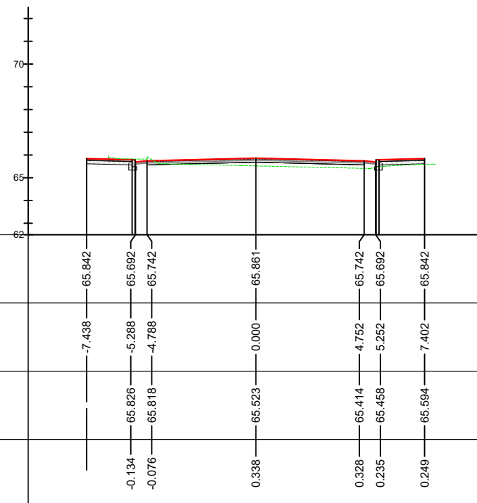
Chainage 30.000 Al - 1
