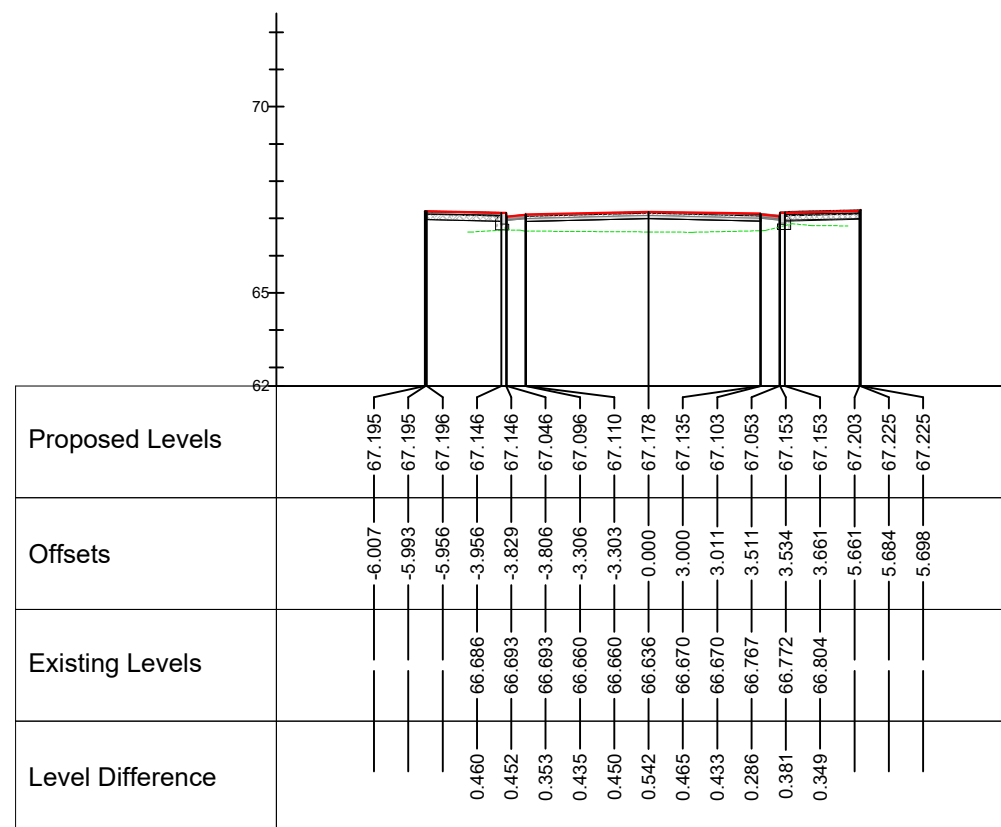
Chainage 25.000 Al-4
