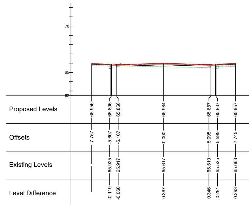
Chainage 35.000 Al - 1
