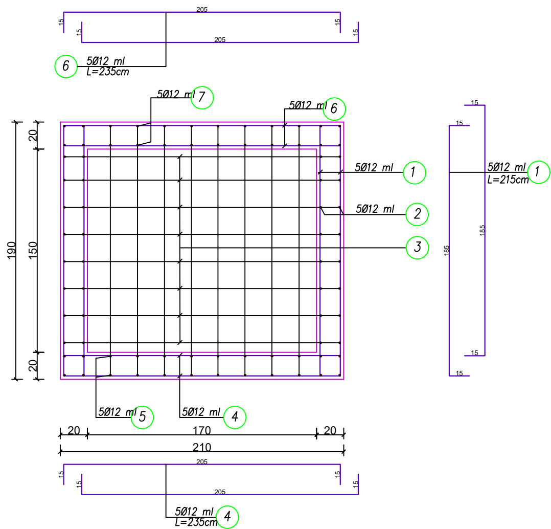
PRERJA A-A SH:1/25
