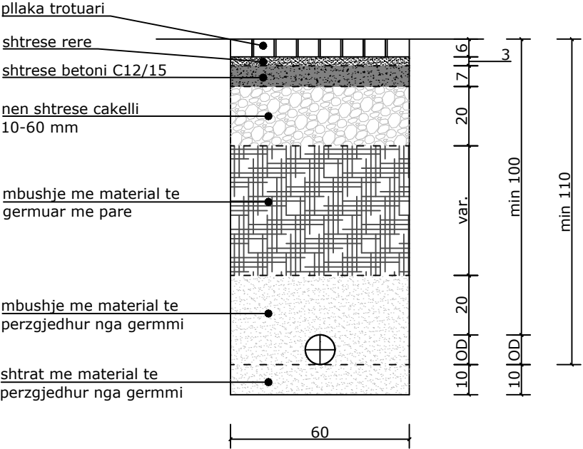
SEKSION TERTHOR TIP I KANALIT PER TROTUAR
