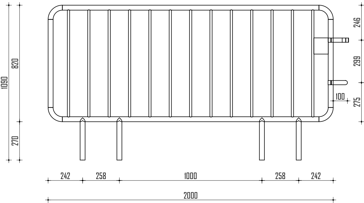
PAMJE BALLORE
