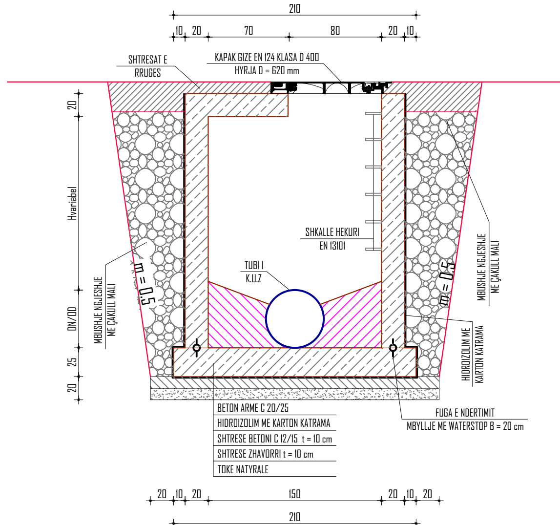
PRERJE TERTHORE
