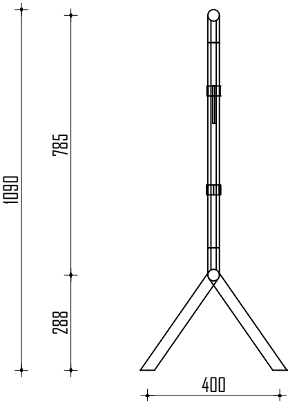
PRERJE TERTHORE
