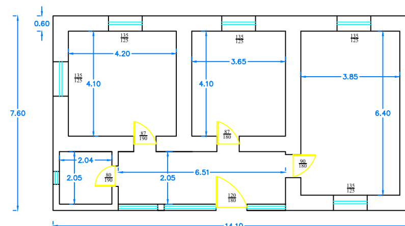
Planimetria e katit 1
