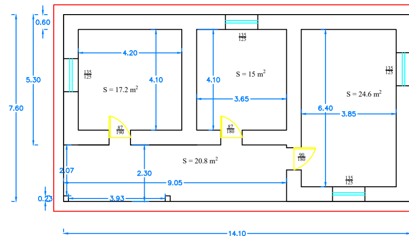
Planimetria e katit 2
