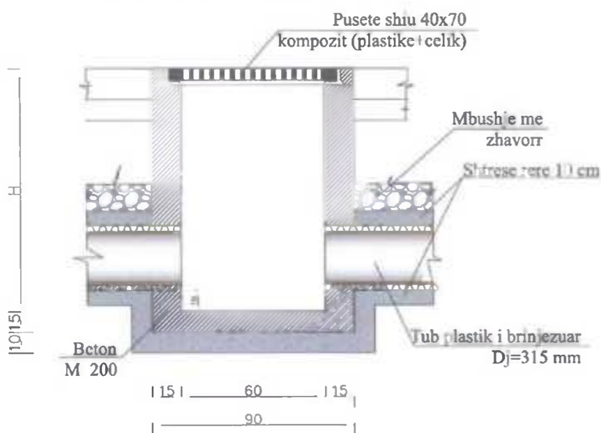
PRERJE A-A SH. 1:20
