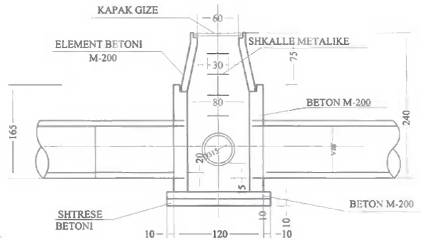
PRERJA 2-2 SHK.1:50
