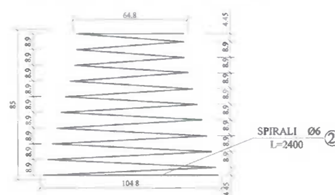
SPIRALI BRENDESHEM SHK.1:20
