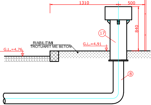
SEKSIONI C-C SHKALLA 1:20
