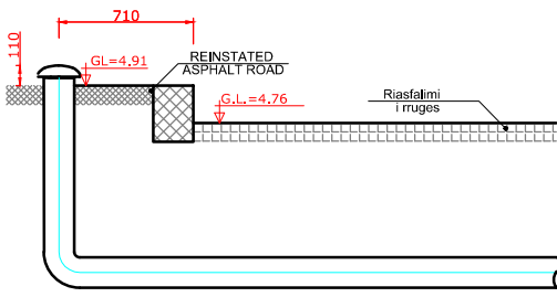
SEKSIONI D-D Scale 1:20
