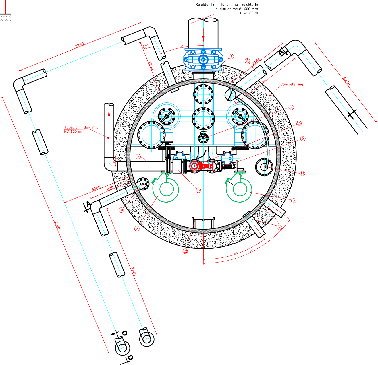
SEKSIONI B-B SHKALLA 1:20
