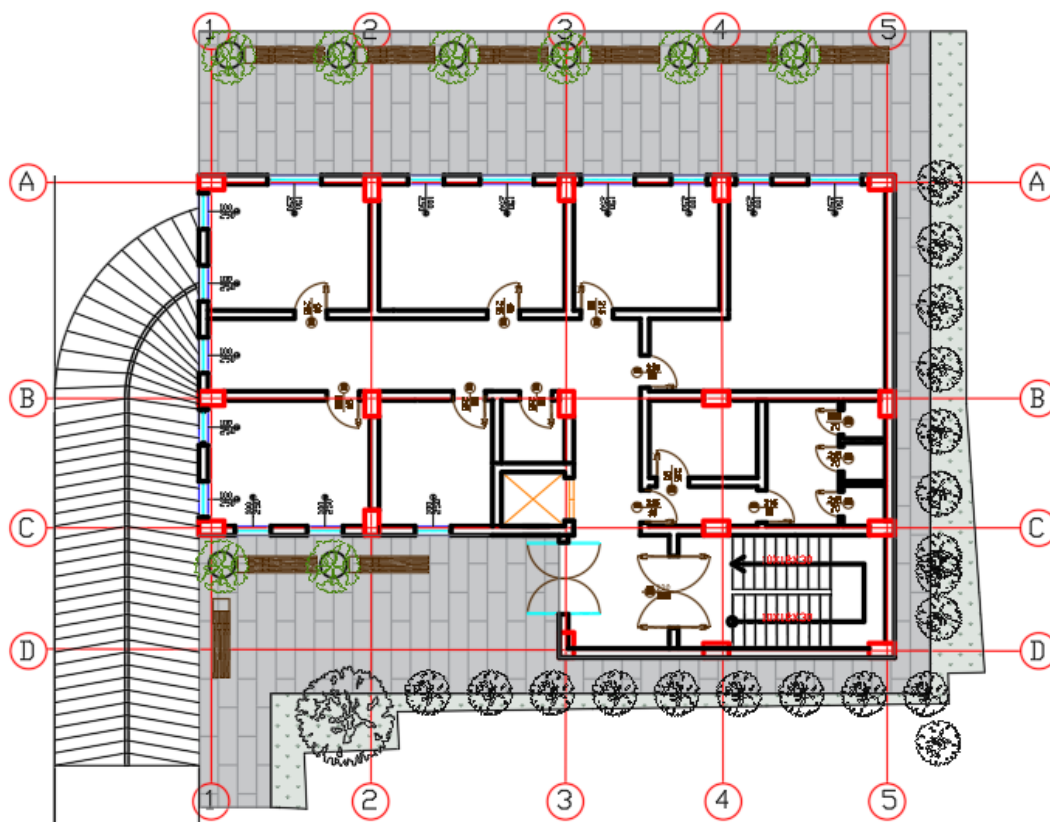
Foto 1 Plani i sistemit te objektit
