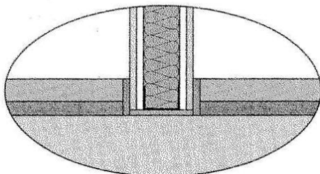
Figura Nr. 5 (detaj i hollesishem i lidhjes ne prejren vertikale)
