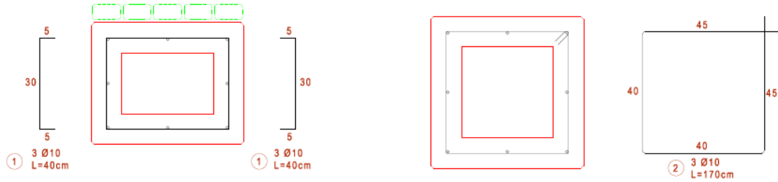
Detaj Armimi i Stolave
