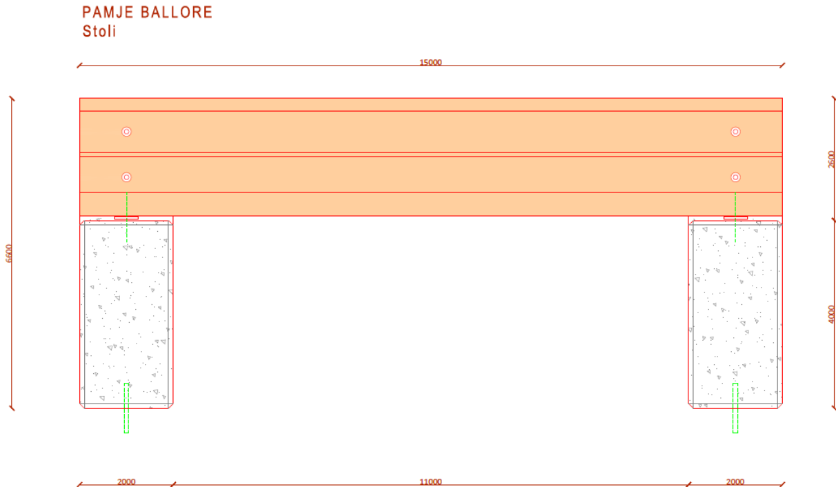
Pamje Ballore e Stolit
