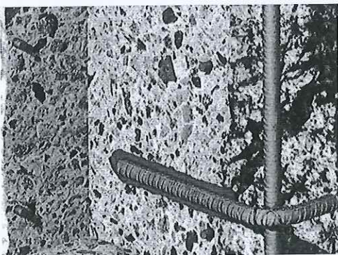
DETAJ I RIPARIMEVE TE MUREVE TE DEMTUARA
